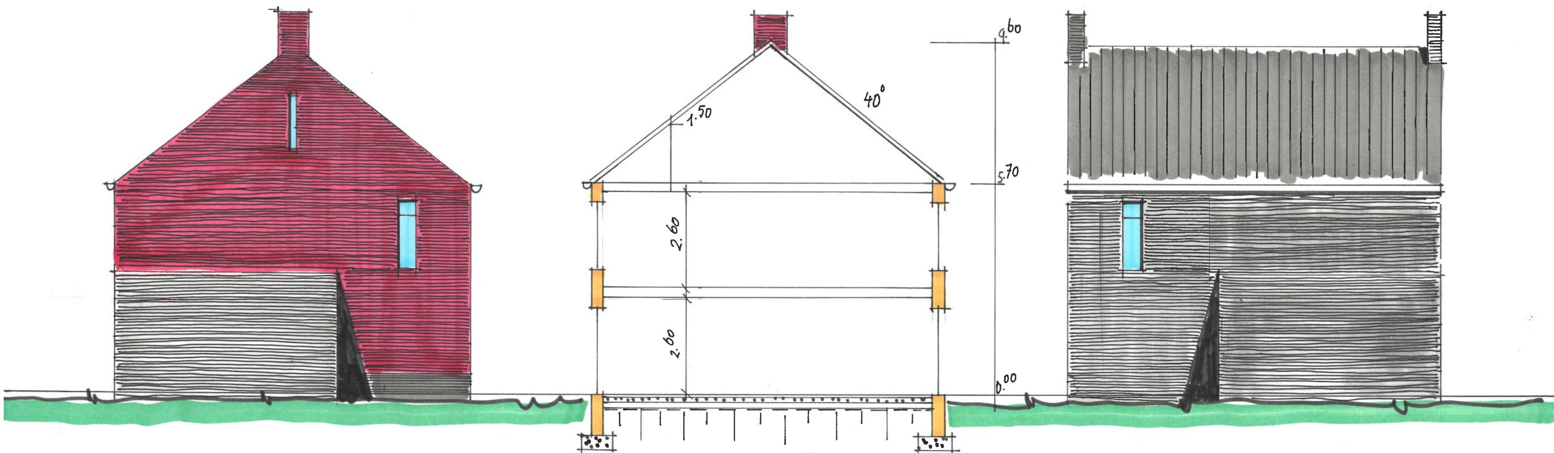
~ LINKER ZYGEVEL ~
