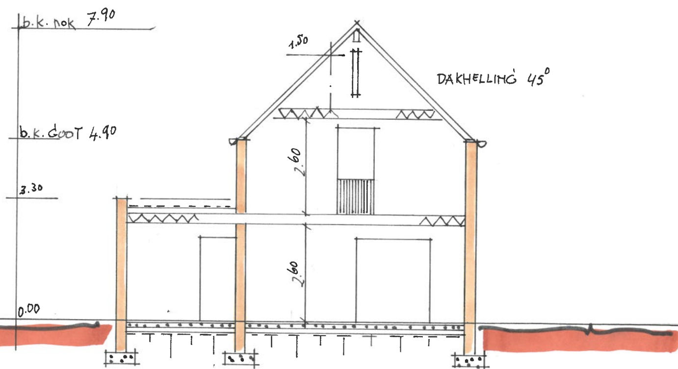
~ DOORSNEDEN ~
